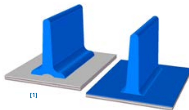
[1] Konwencjonalny zabierak [2] Higieniczny zabierak bez stopki
